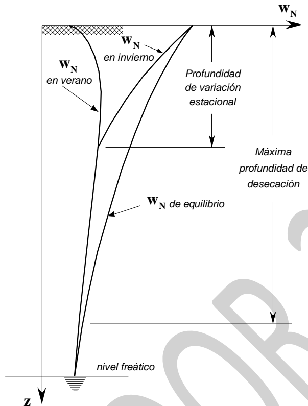
Figura H.9.1-2 – Profundidad de la zona activa y variaciones estacionales de la humedad
